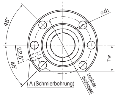
Bohrbild 1 (Baugröße EBC1605 bis 3210)
