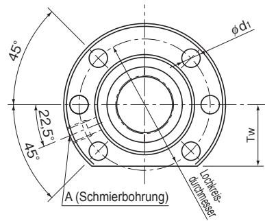
Bohrbild 1 (Baugröße EPC1605 bis 3210)
